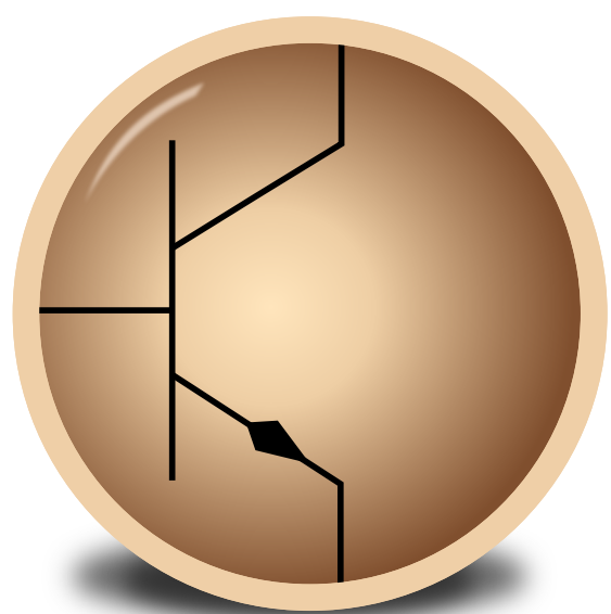
eSim
