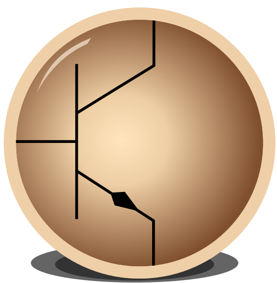
eSim
