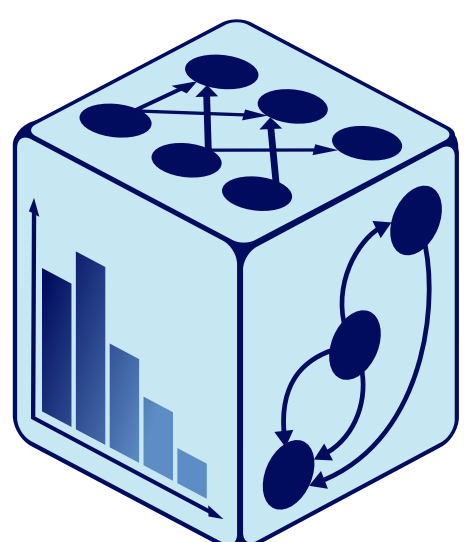
OR-Tools
