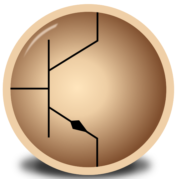
eSim
